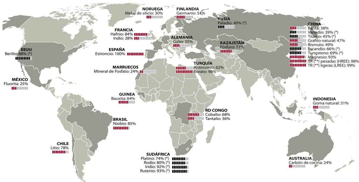
Figura 2. Principales proveedores de la Unión Europea de Materias Primas Críticas en 2020 (Critical Raw Materials o CRM, en porcentaje sobre el total)
